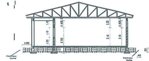
COUPE A-A SECTION A-A
