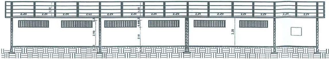
COUPE B-B - SECTION B-B
